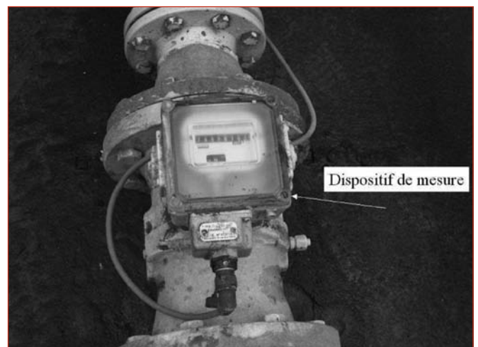
Figure 2: Compteur à gaz.
